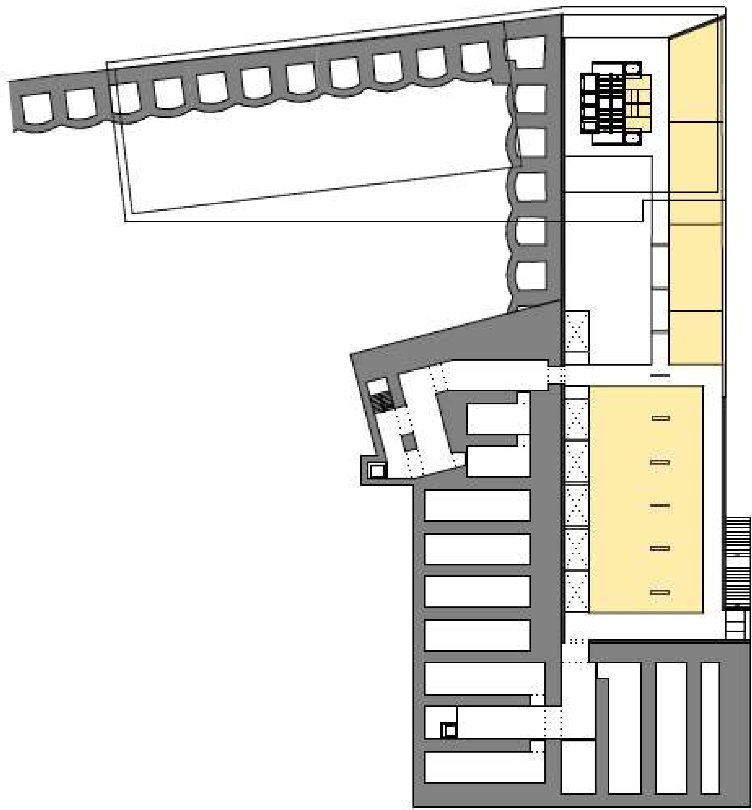
FUNDAMENTE / SOCKELGESCHOSS 720,83 m 2 NUF
