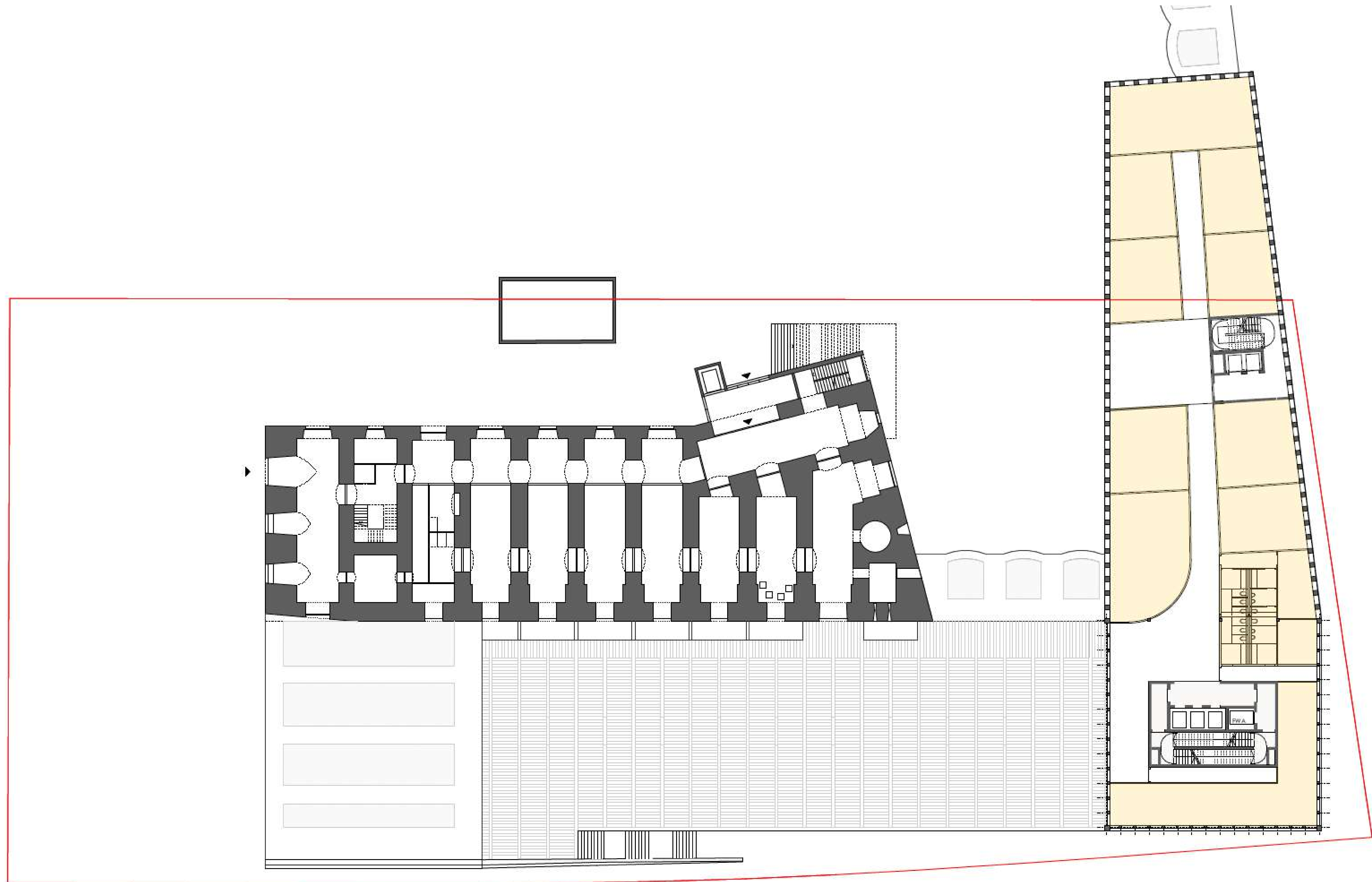
Grundriss Erdgeschoss – Hochschul-Campus
