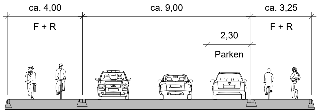
Schnitt A-A
