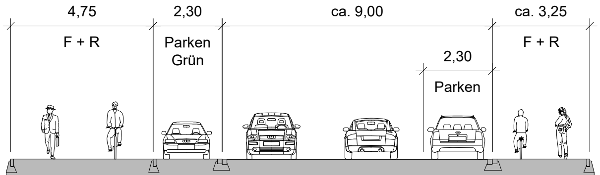
Schnitt B-B
