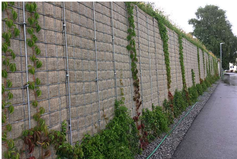
Variante 5, Gabionenwand
