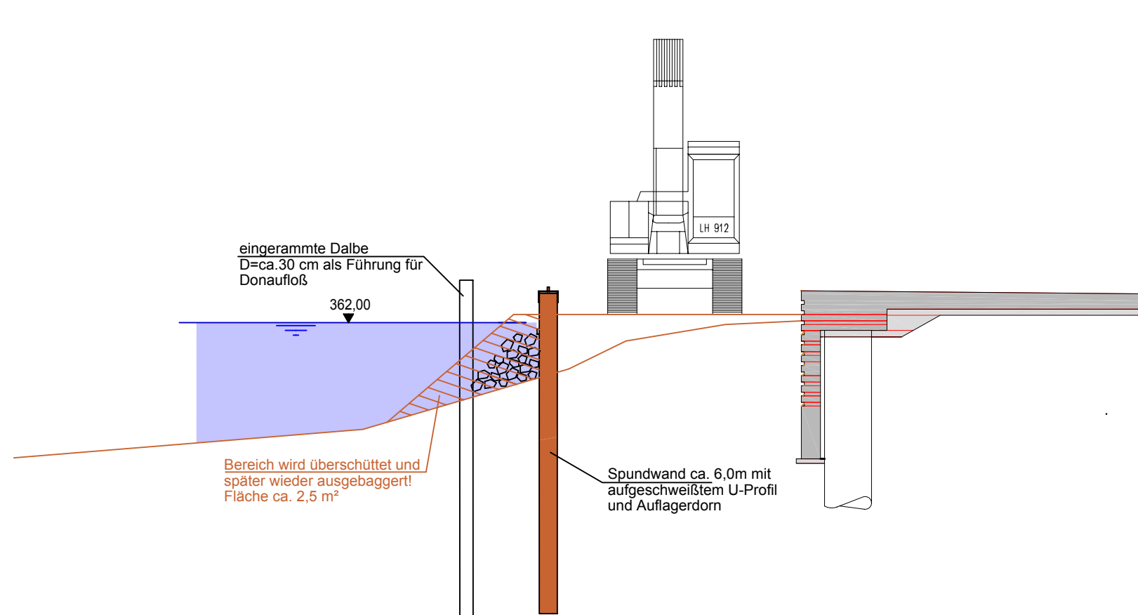
Schnitt Bauzustand M=1:100
