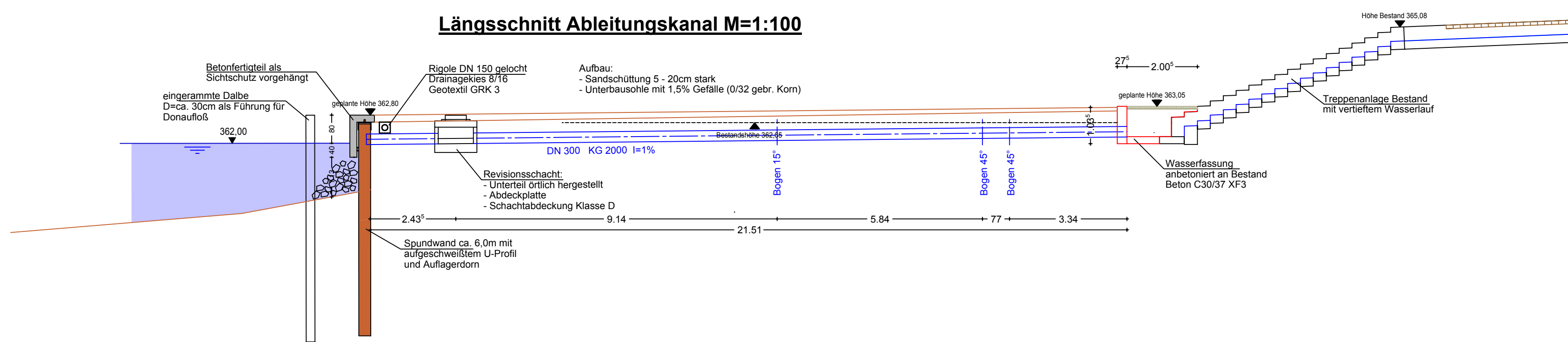
Längsschnitt Ableitungskanal M=1:100
