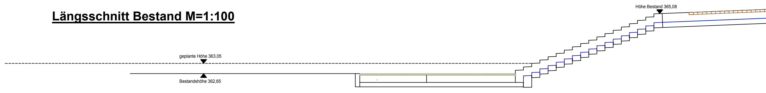
Längsschnitt Bestand M=1:100
