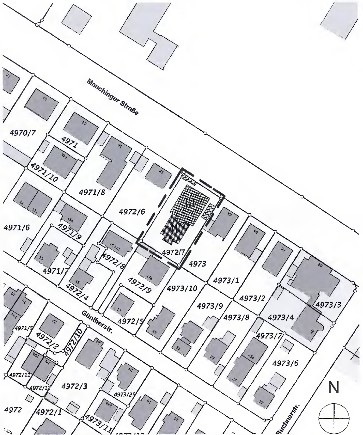
Lageplan
